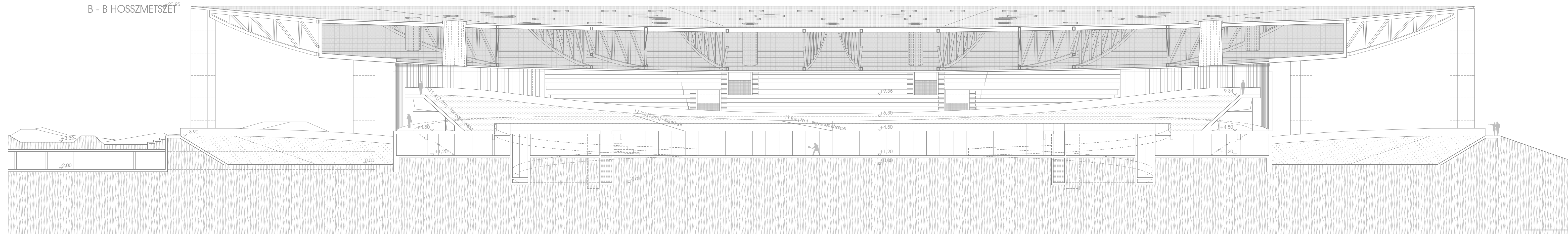
B - B HOSSZMETSZÉT
